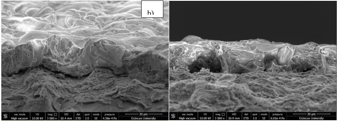
Şekil 2.3. a) \text{TiO}_2 ilavesiz elektrolit içerisinde büyütülen kaplamaya ait kesit görüntüsü b) \text{TiO}_2 ilaveli elektrolit içerisinde büyütülen kaplamaya ait kesit görüntüsü
