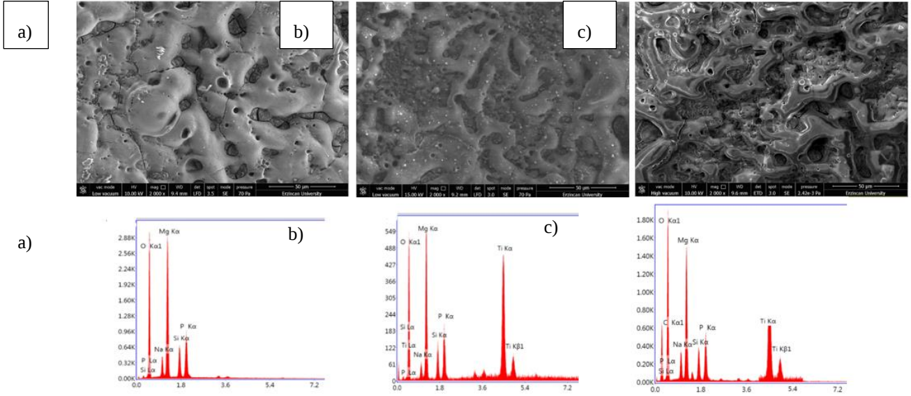
Şekil 2.1. a) \text{TiO}_2 ilavesiz elektrolit içerisinde büyütülen kaplamanın SEM görüntüsü ve EDX analizi b) \text{TiO}_2 ilaveli elektrolit içerisinde büyütülen kaplamanın SEM görüntüsü ve EDX analizi c) \text{TiO}_2 ve C ilaveli elektrolit içerisinde büyütülen kaplamanın SEM görüntüsü ve EDX analizi
