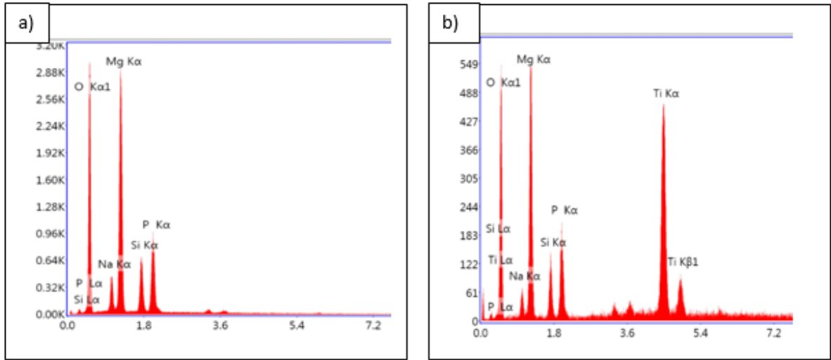
Şekil 2.2. a) \text{TiO}_2 ilavesiz elektrolit içerisinde büyütülen kaplamaya ait EDX ve b) \text{TiO}_2 ilaveli elektrolit içerisinde büyütülen kaplamaya ait EDX
