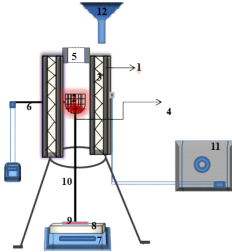
Şekil 1. Deneysel sabit yatak yakma sistemi: 1. Refrakter tuğla; 2. Sepet; 3. Direnç teli; 4. Biyokütle; 5. Fırın kapağı; 6. Termocift; 7. Terazi; 8. Destek; 9. Ayna; 10. Sepet çubuğu; 11. Gerilim değiştirici; 12. Besleme hunisi
