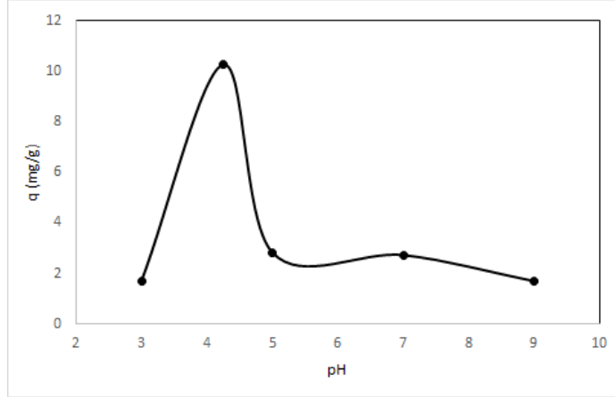
Şekil 6. pH'nın adsorpsiyon kapasitesine etkisi [25°C, [RB]=50mg/L, 0,5 mg/mL NaAlg/HPMC]
