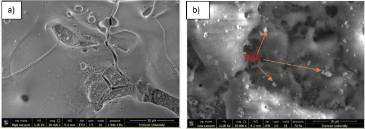
Şekil 2.1. a) \text{TiO}_2 ilavesiz elektrolit içerisinde büyütülen kaplamanın SEM görüntüsü ve b) \text{TiO}_2 ilaveli elektrolit içerisinde büyütülen kaplamanın SEM görüntüsü
