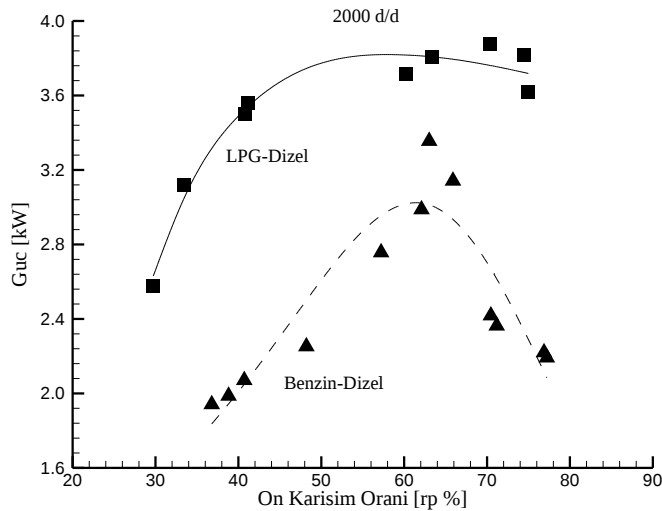
Şekil 3. Değişken r_p Değerlerine Göre Güç Değişimi
