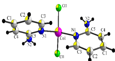
Fig.1. l'unité asymétrique de [\text{Co}(\text{C}_5\text{H}_6\text{N}_2)_2]\text{Cl}_2
