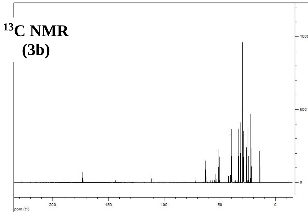
Şekil 2. Tri-katyonik yüzey aktif maddelerin ^1\text{H} NMR ile ^{13}\text{C} NMR spektrumları
